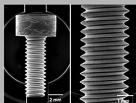
●温室塑性加工(転造)によるM3ネジ
