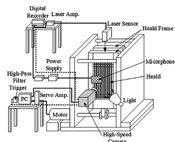
開口シミュレータを用いた織機構成部品の解析
