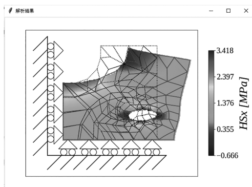
アイソレート要素法による解析結果
