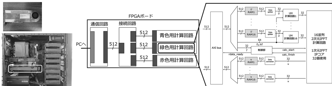
ホログラフィ専用計算機の外観と計算回路の構成。
