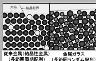
●従来の結晶性金属と金属ガラスの原子配列の比較
