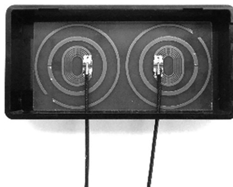
(b)ローカル5G用平面アンテナ FMSP-L5G-RxW 寸法(mm) : 34×34×0.4
