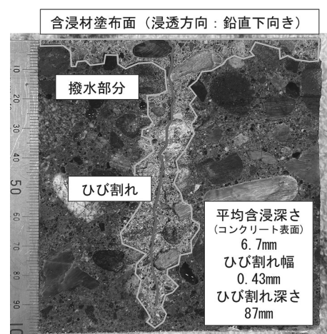
写真2 撥水性含浸材を用いた ひび割れ補修の試み
