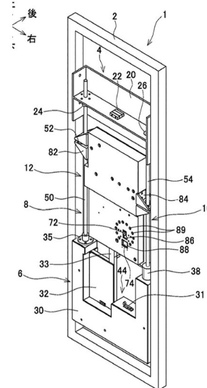
図2：検査機器移動機
