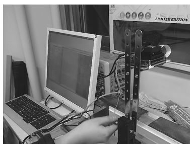
画像処理によるレール遊間測定
