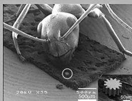
●超塑性形成による金属ガラス製マイクロ歯車
