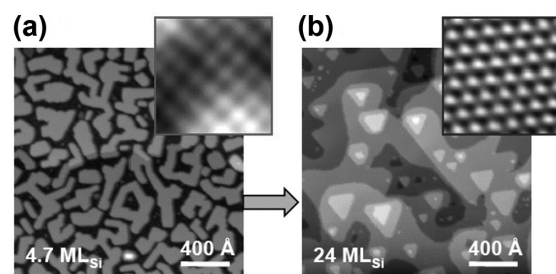
図1 Si (111) 7 \times 7 上のBi超薄膜の構造変態前(a)と後(b)のSTM像。挿入図：BP膜(a)とHEX膜(b)の高分解能像 ( 3 \times 3 \text{ nm}^2 )。
