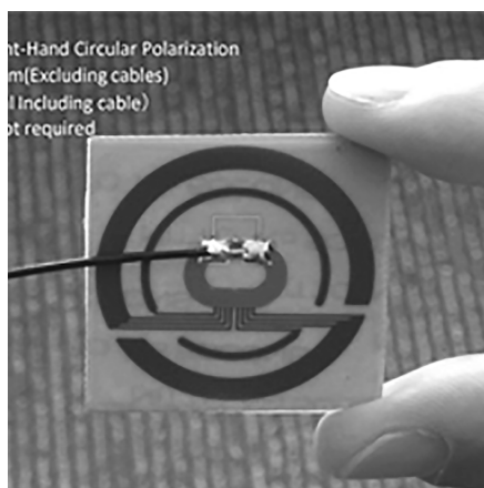
(a)みちびき対応アンテナ FMSP-QZSS-Q55 寸法(mm)/重量(g) : 34×34×0.4/ 約1.5
